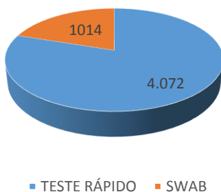
Quantidade de testes realizados por tipo de amostragem
